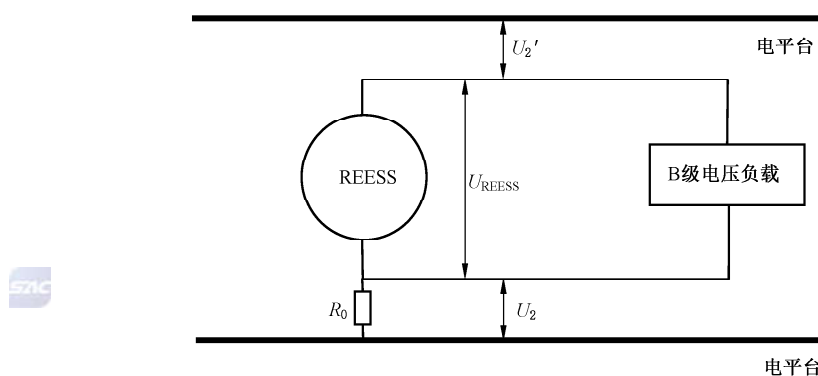
图 5 绝缘电阻测量步骤 c)
